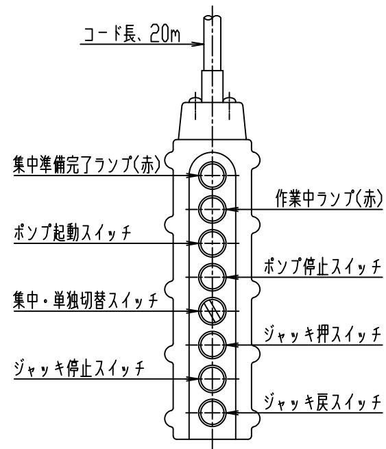
遠隔操作手元スイッチ
