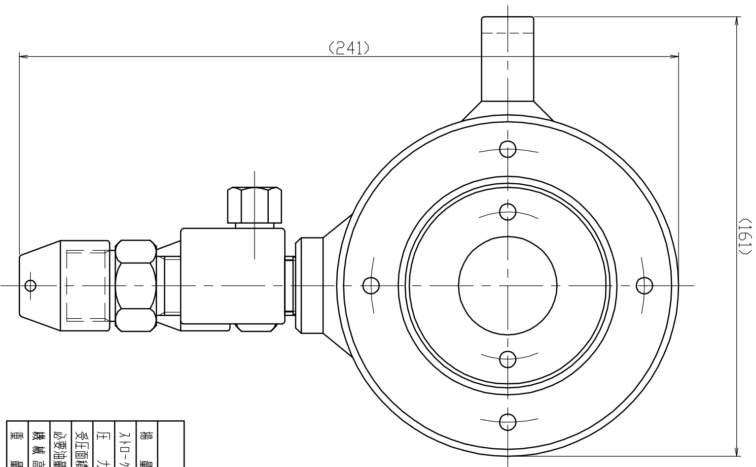
Y方向矢視図
