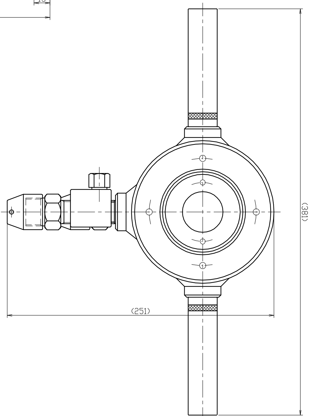
Y方向矢視図
