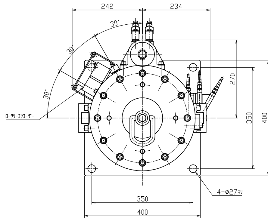
P方向矢視図
